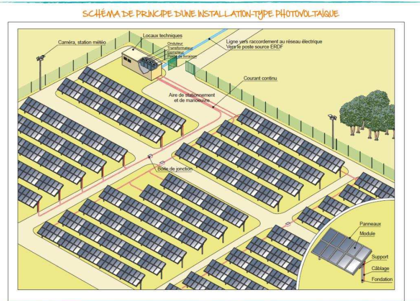
Figure 2 : Schéma de principe d'une installation-type photovoltaïque
